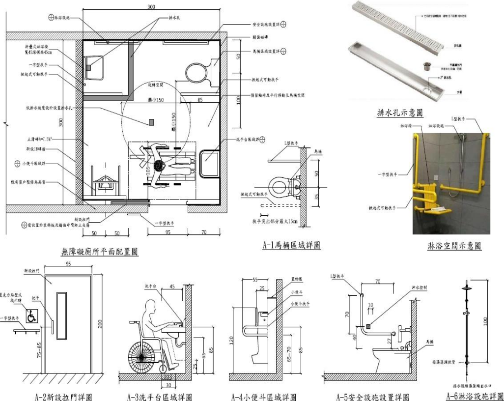
無障礙廁所規劃設計圖
