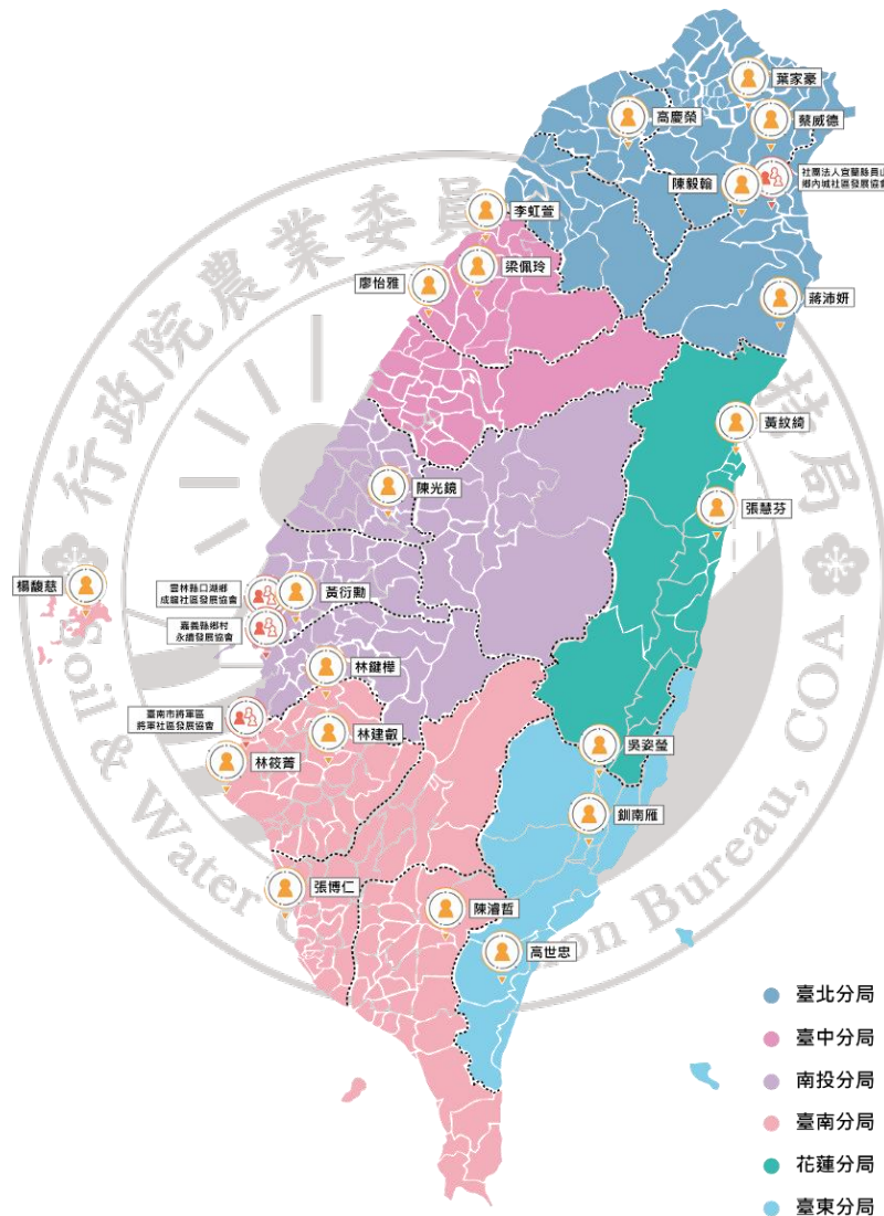
圖 2-7 全台優秀青年、團隊分布圖
